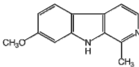
Harmina 7-metoxi-1-metil-b-carbolina, C_{13}H_{12}N_2O
