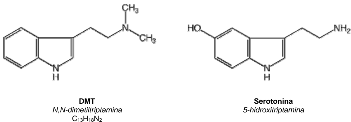
Fig. 15: Estruturas químicas da DMT e da Serotonina.
