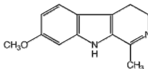
Harmalina 3,4-dihidro-7-metoxi-1-metil-b-carbolina, C_{13}H_{14}N_2O
